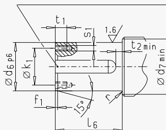
Arbeitsmaschinenwelle Driven machine shaft Arbre de la machine de travail
