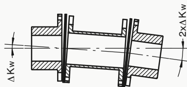
Bild / Figure 3.2 Winkelversatz Angular Misalignment Déviation angulaire
