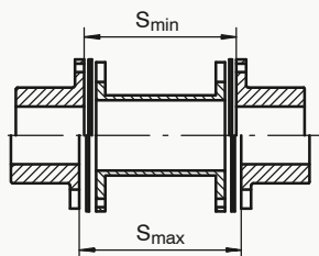
Bild / Figure 3.1 Axialversatz Axial Movement (End float) Déplacement axial
