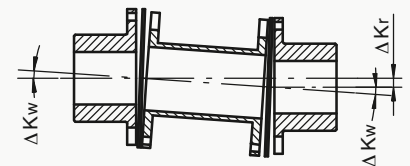
Bild / Figure 3.3 Radialversatz Radial Misalignment Désalignement radial
