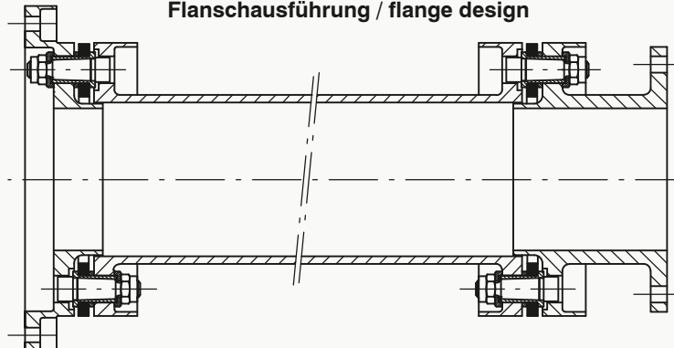
Flanschausführung / flange design
