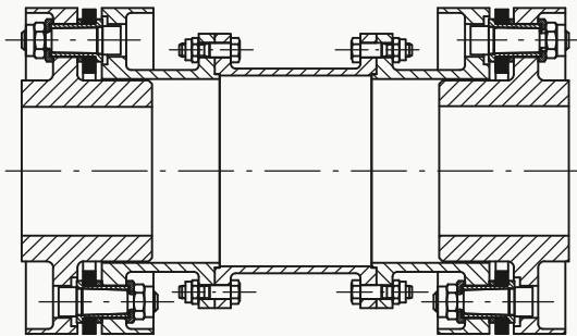
Ausführung / Type BVB
